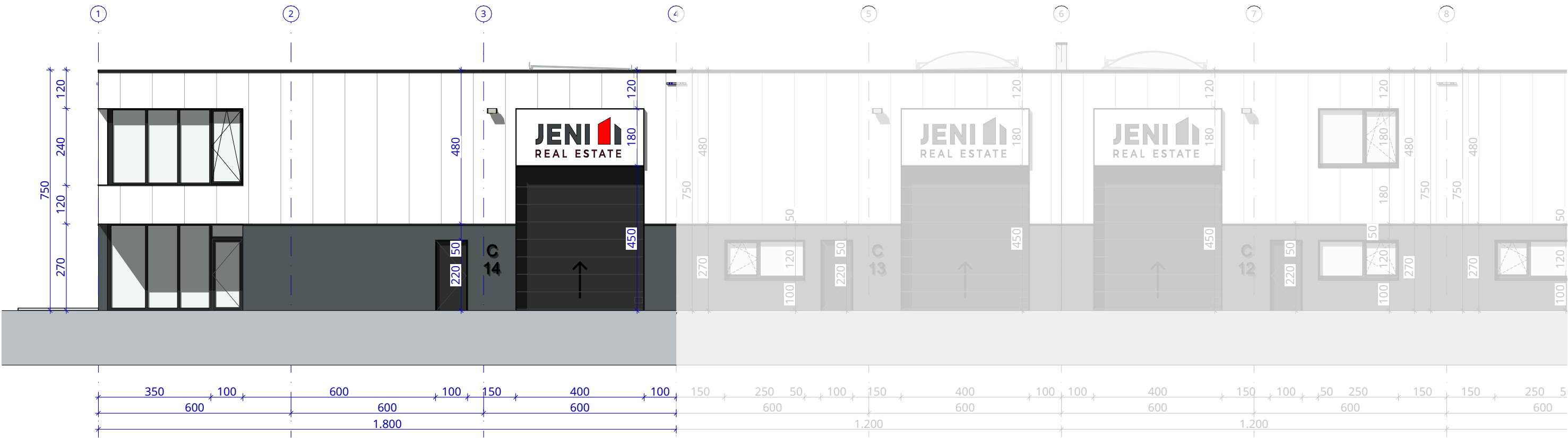
zuidgevel
